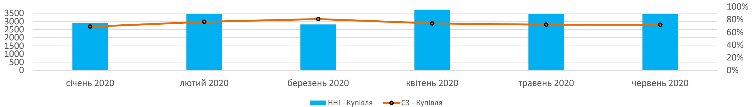
Індекси концентрації ринку (РДН БуОс купівля)
