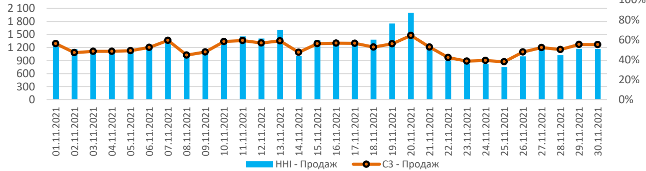
Індекси концентрації ринку (РДН БуОс продаж)
