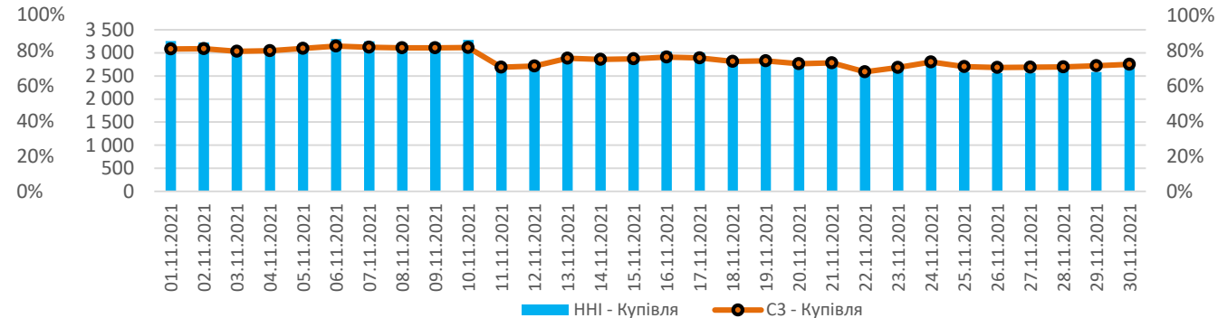
Індекси концентрації ринку (РДН БуОс купівля)
